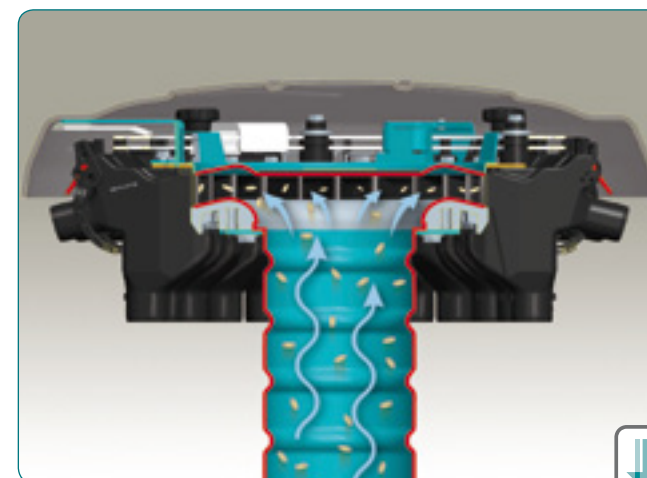
Dozowanie pneumatyczne w 100% SULKY
