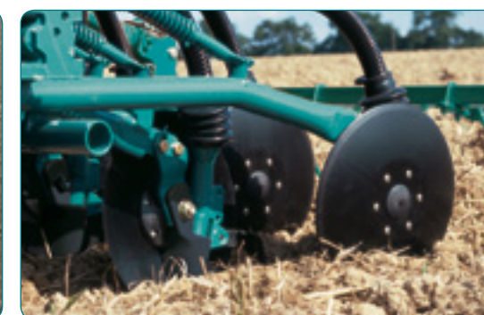
Redlice stopkowe UNISOC 2R lub redlice talerzowe UNIDISC
