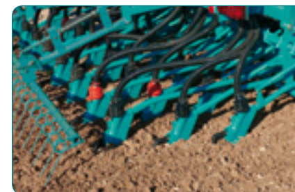
Redlice stopkowe UNISOC 3R lub redlice talerzowe UNIDISC
