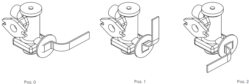
Rys. 9 Ręczny regulator siły hamowania przyczepy T-677
