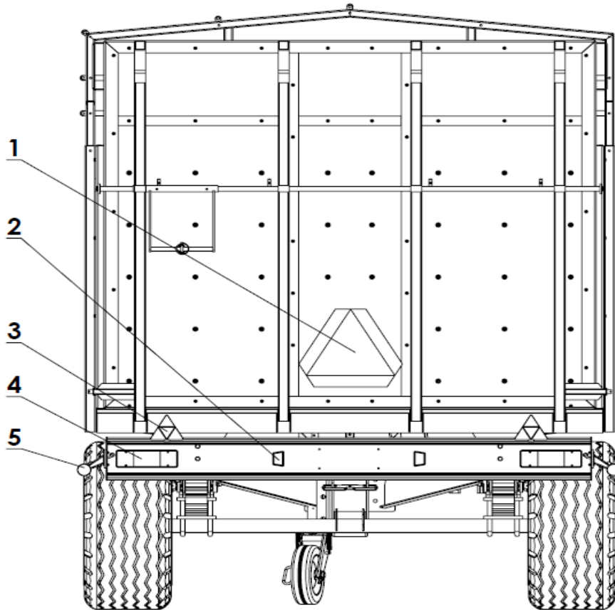
Rys. 1. Przyczepa T-678 (widok z tyłu)
