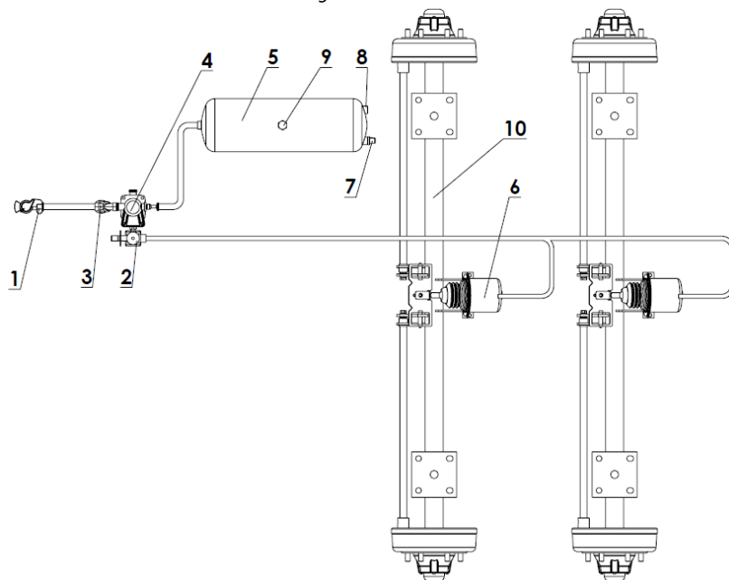
Rys. 7. Schemat instalacji pneumatycznej dwuprzewodowej.
