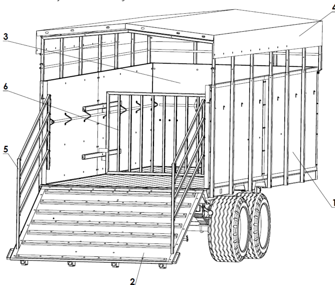
Rys. 5. Skrzynia ładunkowa.
