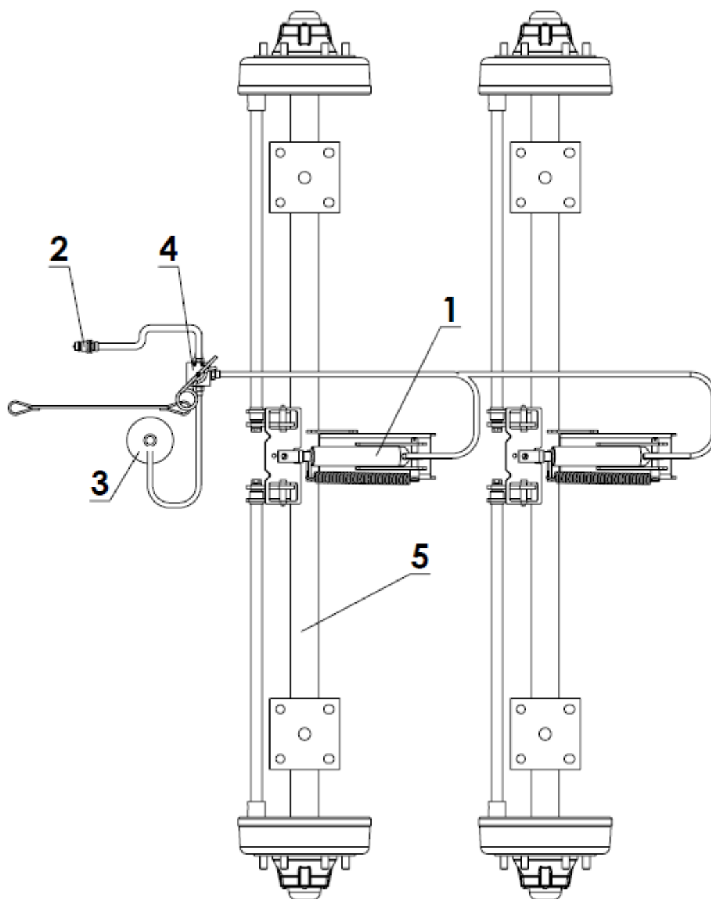
Rys. 8. Schemat instalacji hydraulicznej.
