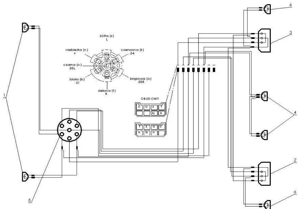
Rys. 10. Schemat instalacji elektrycznej przyczepy.
