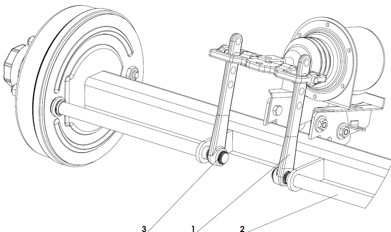
Rys. 13. Elementy regulacji hamulców.
