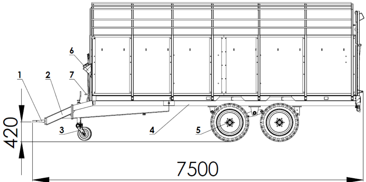
Rys. 2. Przyczepa T-678 (widok z boku).
