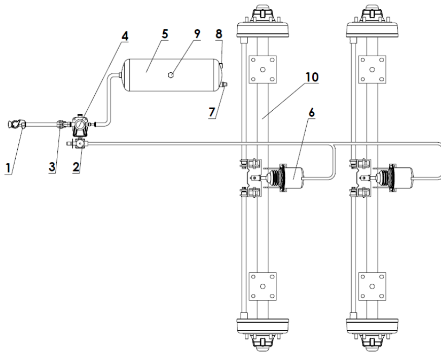
Rys. 6. Schemat instalacji pneumatycznej jedнопrzewodowej.
