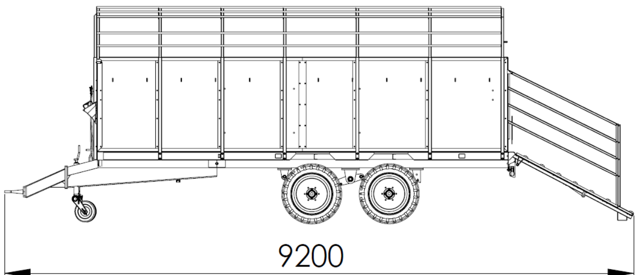
Rys. 3 Przyczepa T-677 z opuszczoną ścianą tylną.
