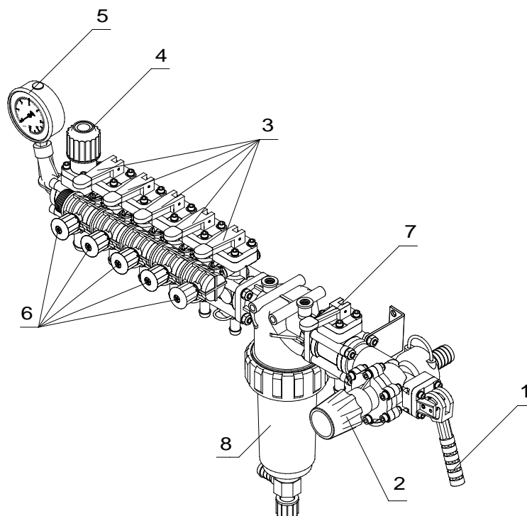
Rysunek 11 Zawór sterujący pięciosekcyjny z kompensacją ciśnienia ARAG
