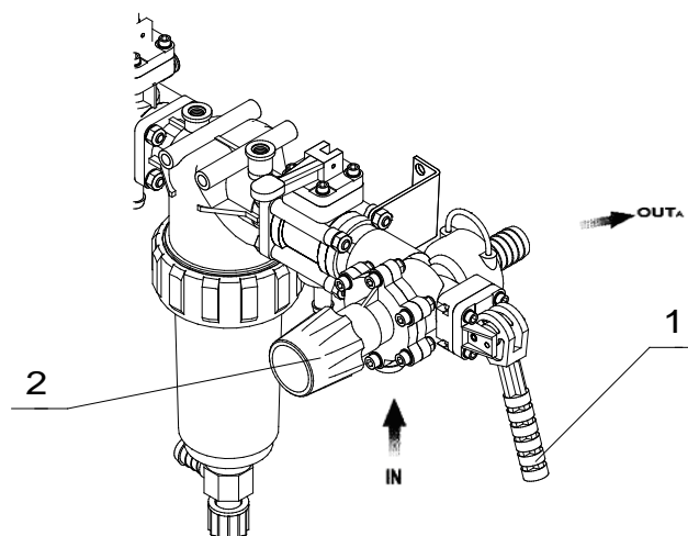
Rysunek 12 Zawór sterujący z kompensacją ciśnienia
