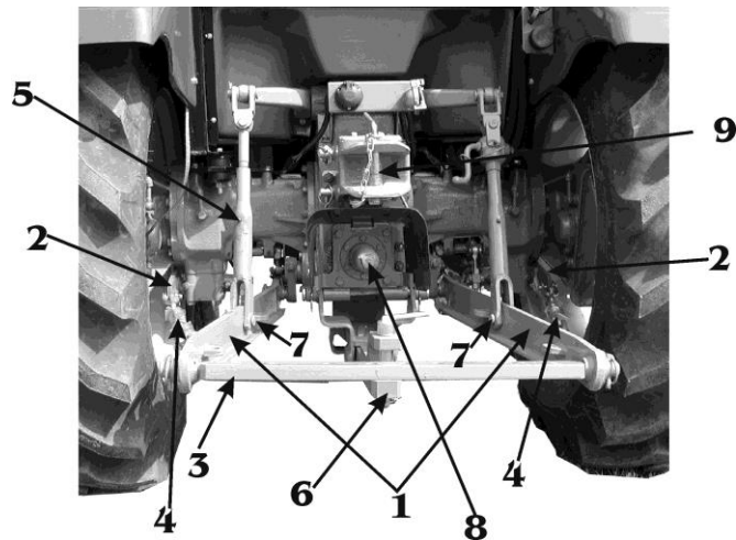
Rysunek 25 Ciągnik przygotowany do współpracy z opryskiwaczem
