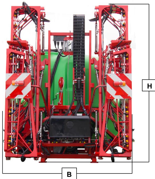
Rysunek 24 Gabaryty w pozycji transportowej
