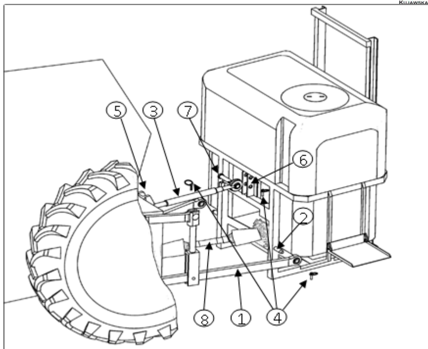
Rysunek 26 Agregowanie ciągnika z opryskiwaczem
