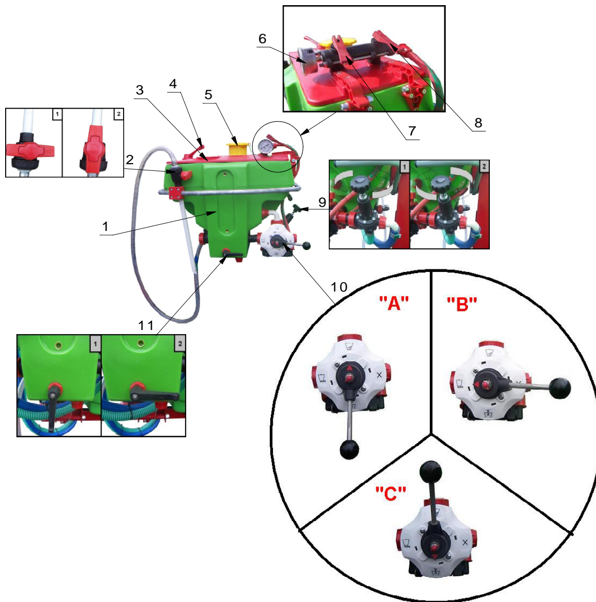
Rysunek 9 Budowa rozwadniacza bocznego POLMAC
