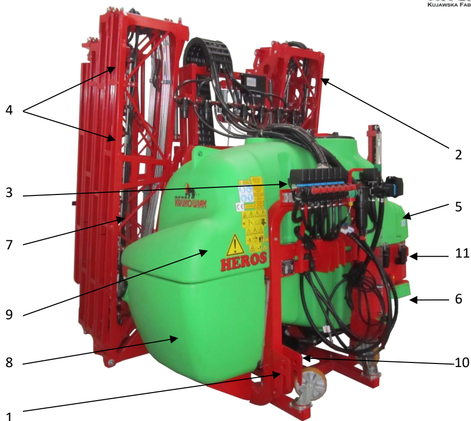
Rysunek 4 Opryskiwacz polowy zawieszany
