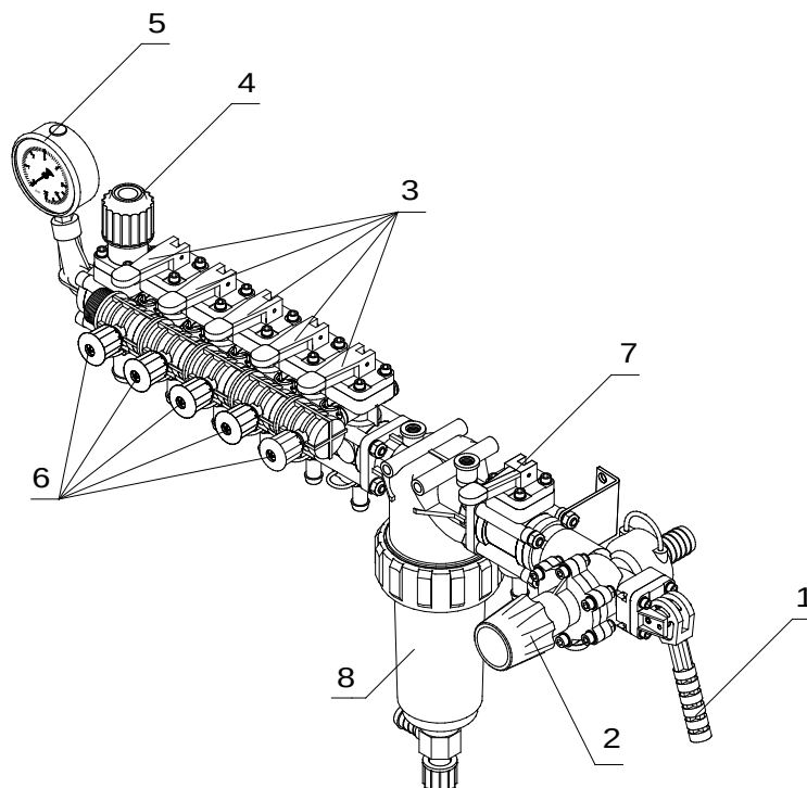
Rysunek 11 Zawór sterujący sześćosekcyjny z kompensacją ciśnienia ARAG
