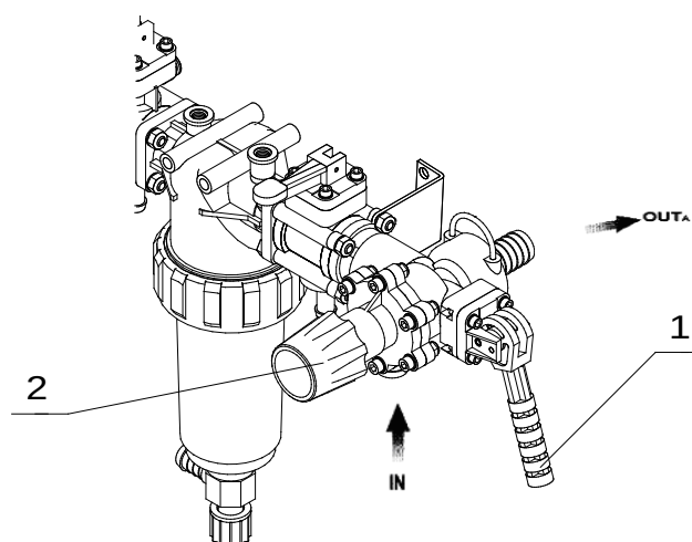
Rysunek 12 Zawór sterujący z kompensacją ciśnienia
