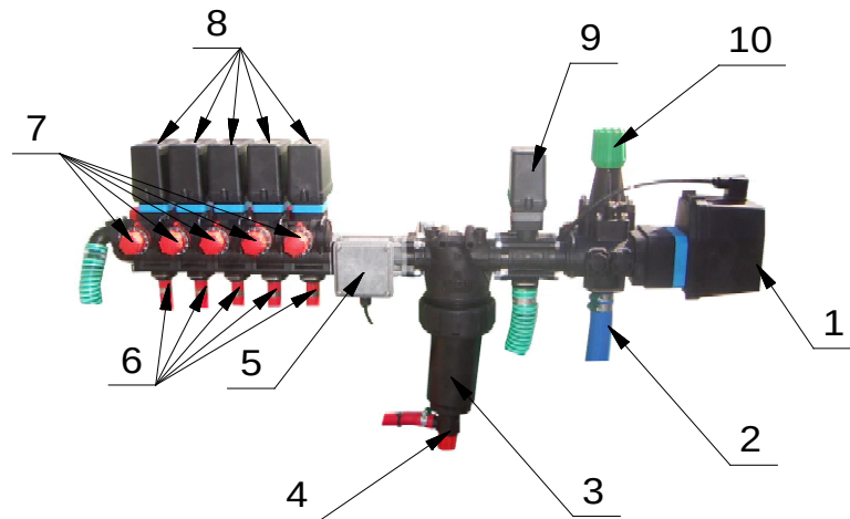
Rysunek 9 Zawór cieczowy sterowany elektrycznie
