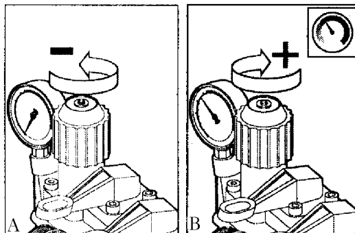
Rysunek 14 (A, B) Zawór ciśnienia proporcjonalnego
