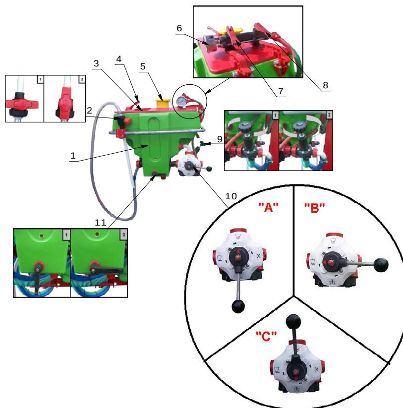
Rysunek 9 Budowa rozwadniacza bocznego POLMAC
