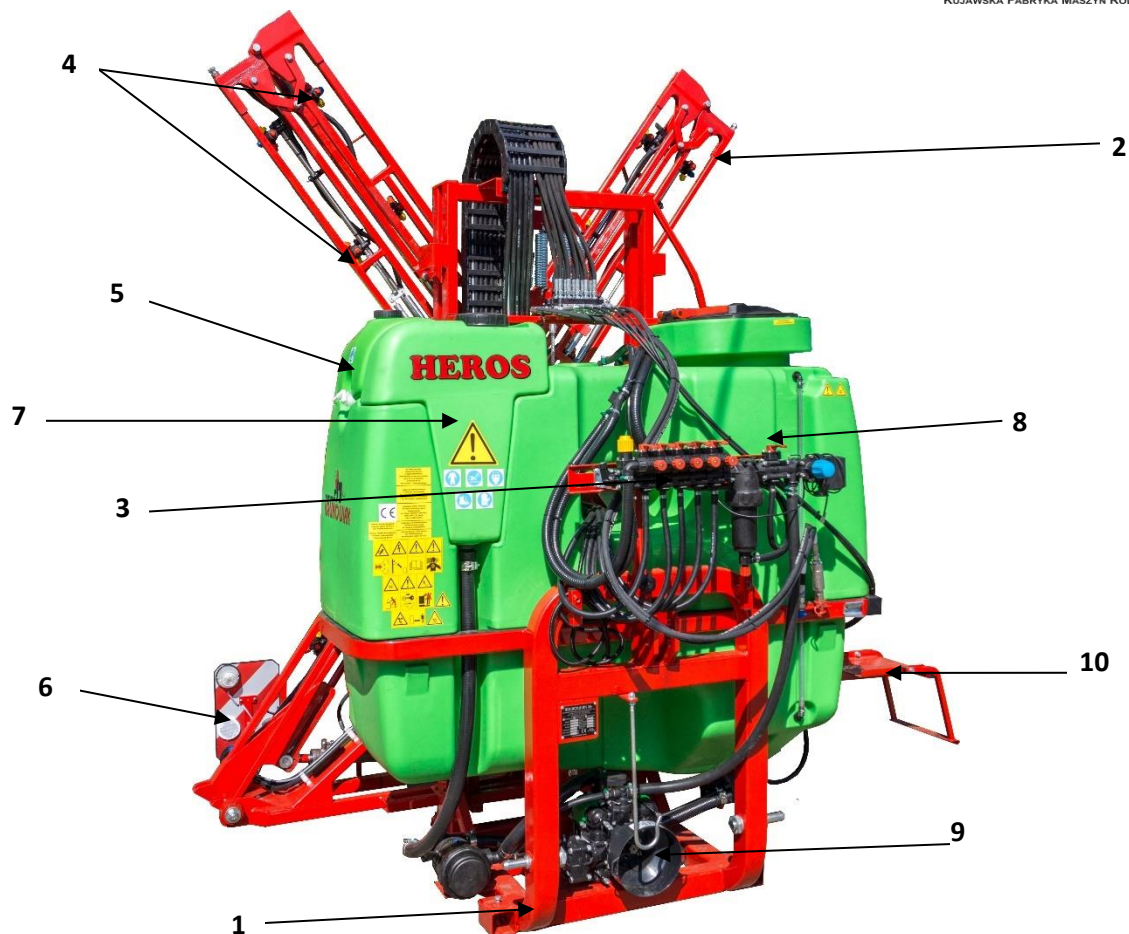
Rysunek 4 Opryskiwacz polowy zawieszany HEROS PHX.
