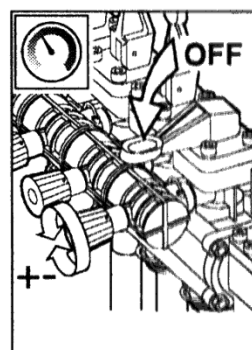
Rysunek 18 Zawór ciśnienia proporcjonalnego
