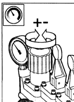
Rysunek 17 Zawór ciśnienia proporcjonalnego
