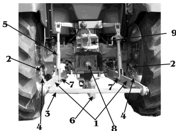
Rysunek 26 Ciągnik przygotowany do współpracy z opryskiwaczem
