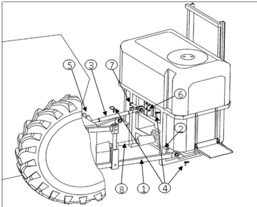
Rysunek 27 Agregowanie ciągnika z opryskiwaczem
