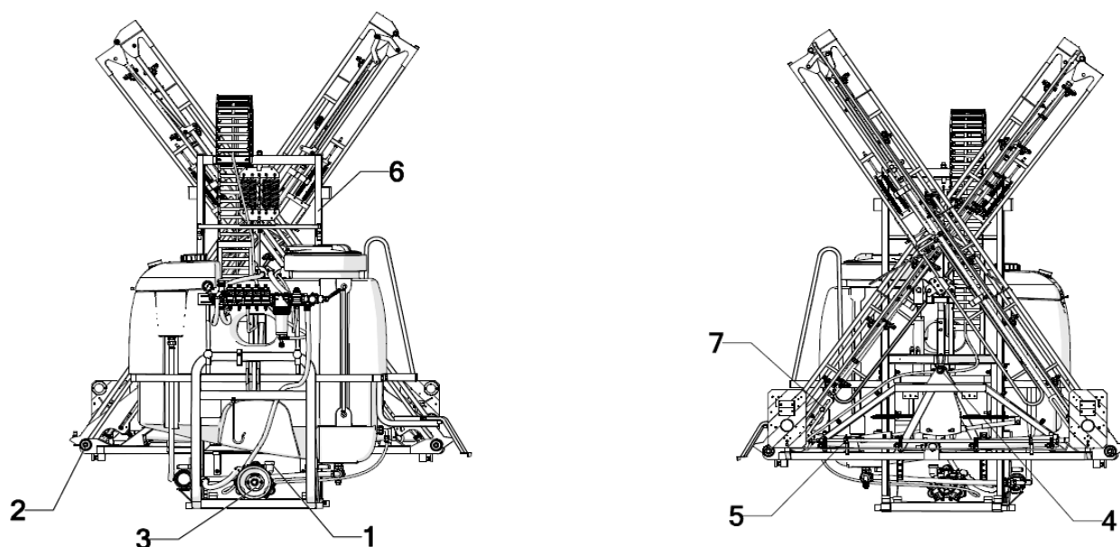
Rysunek 10 Punkty smarowania opryskiwacza HEROS PHX.
