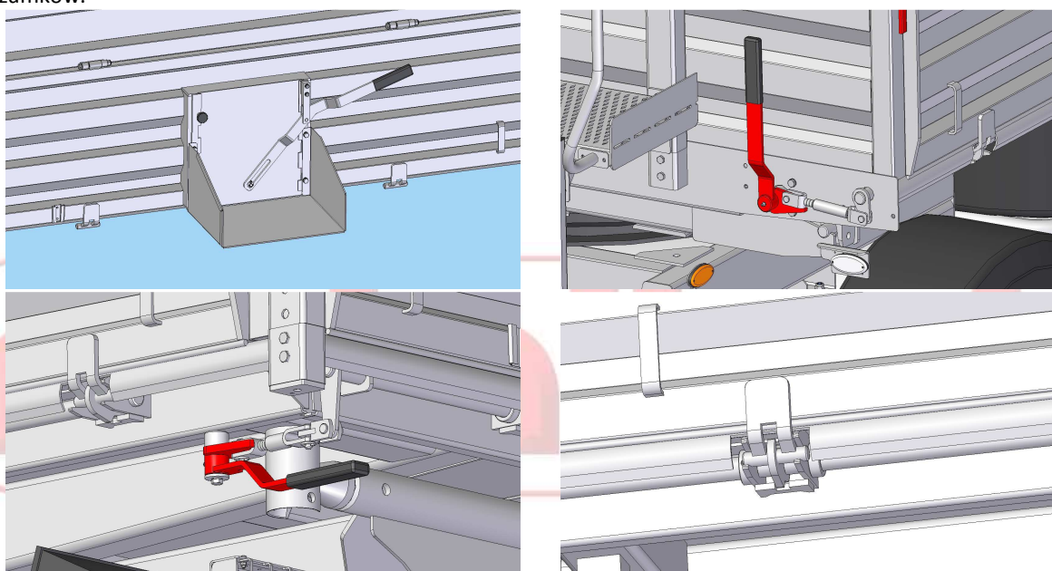
Rys. 7. Okno zsypane i zamki burt skrzyni ładunkowej.
