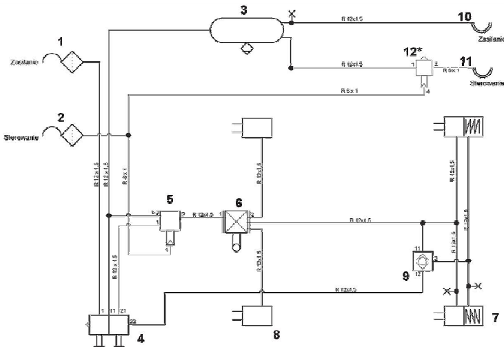
Rys. 3. Schemat pneumatycznej instalacji hamulcowej 1- złącze przewodów z filtrem, zasilenie, 2- złącze przewodów z filtrem, sterowanie, 3- zbiornik powietrza, 4- zawór luzująco-parkujący, 5- zawór hamulcowy przyczepy, 6- automatyczny regulator siły hamowania, 7- siłownik hamulcowy, membrano-sprężynowy, 8- siłownik hamulcowy membranowy, 9- zawór 2/3 drogowy, 10- złącze przewodów z zaworem, zasilenie, 11- złącze przewodów z zaworem, sterowanie, 12- zawór przełącznikowy
