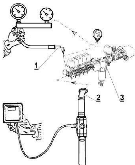
Rys. 59. Pomiar kontrolny przepływu cieczy i manometru:
