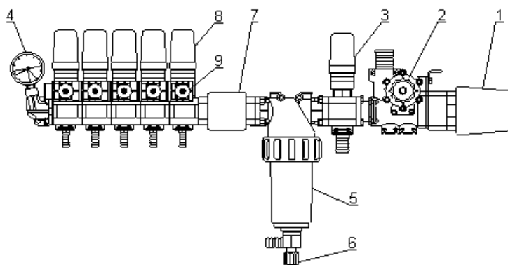
Rys. 25. Elektrozawór kpl.
