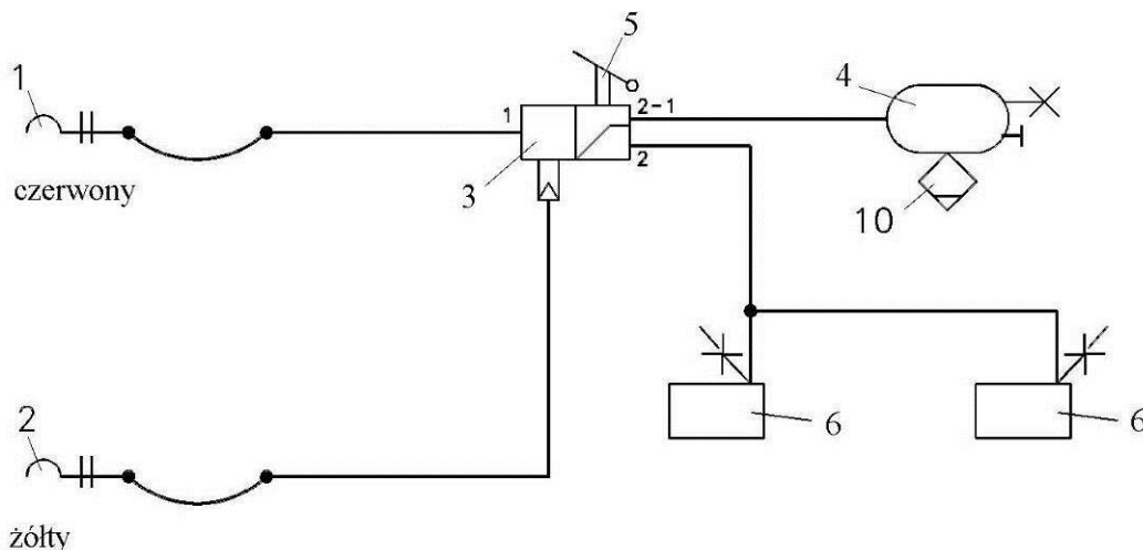
Rys. 45. Układ pneumatyczny opryskiwacza w wersji podstawowej (bez pneumatycznego zawieszenia)
