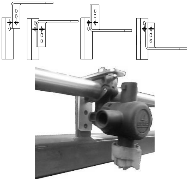
Rys. 37 Widok elementów pozycjonujących rury układu opryskowego
