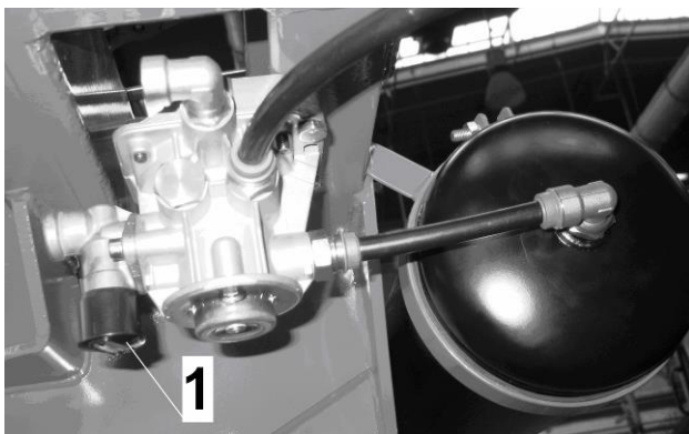
Rys. 43. Zawór hamulcowy opryskiwacza:
