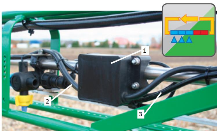
Rys. 39 Elektrozawór sterujący otwarciem dyszy w EDS
