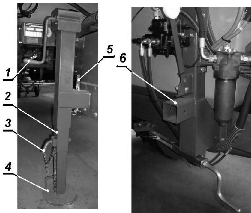
Rys. 6 Podpora przy dyszlu śledzącym.
