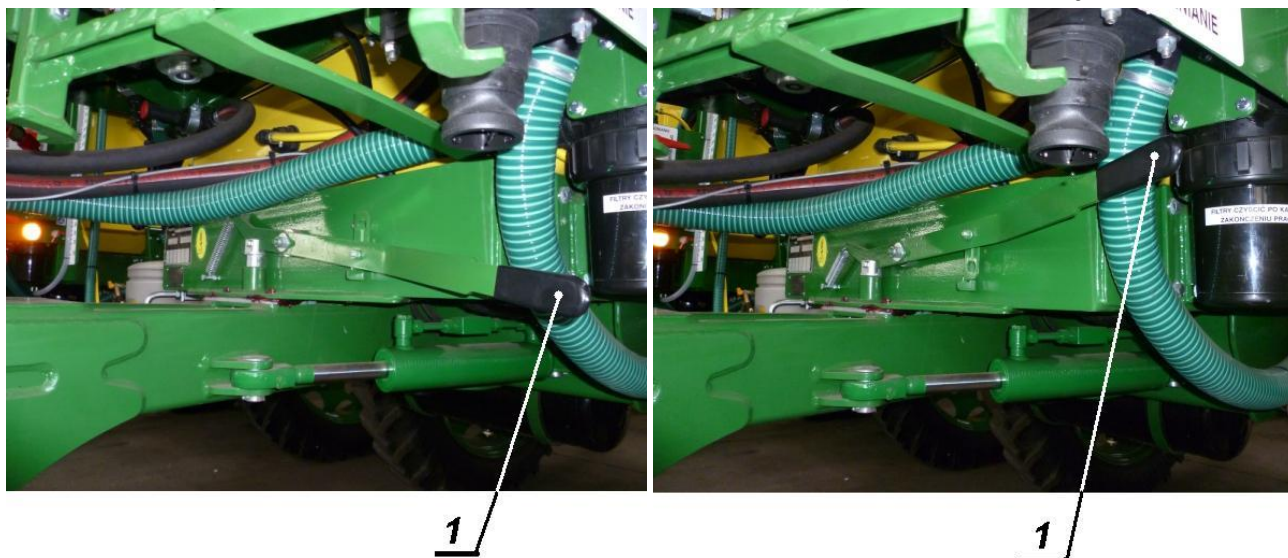
Rys. 54. Blokada dyszla śledzącego
