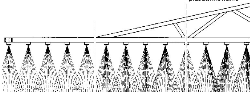
Rys. 58. Widok oprysku belką polowa: z nowymi, zablokowanymi i uszkodzonymi rozpylaczami
