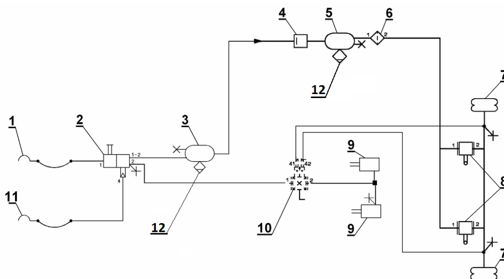
Rys. 44. Układ pneumatyczny opryskiwacza z pneumatycznym zawieszeniem (opcja)
