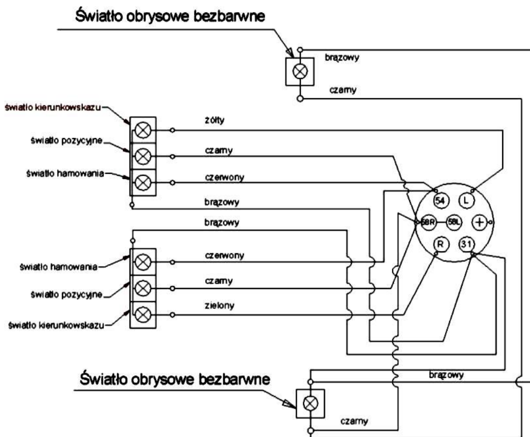
Rys. 60 Schemat instalacji elektrycznej (12V)
