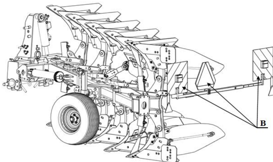
Rysunek:6 Transport
