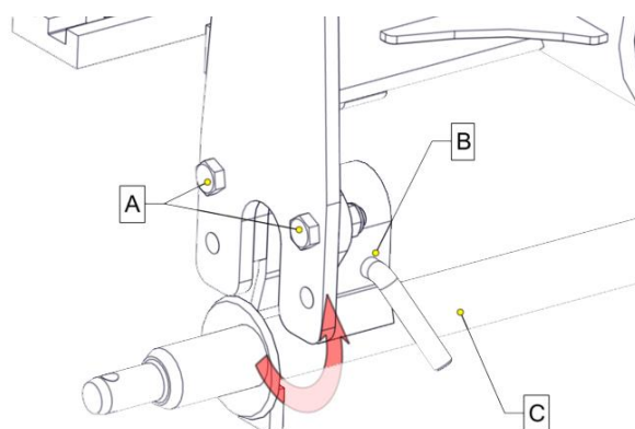
Rysunek:7 Oś zawieszenia
