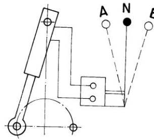
Rysunek:17 Obrót
