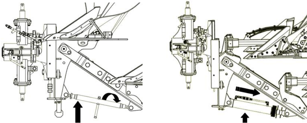
Rysunek:20 Regulacja
