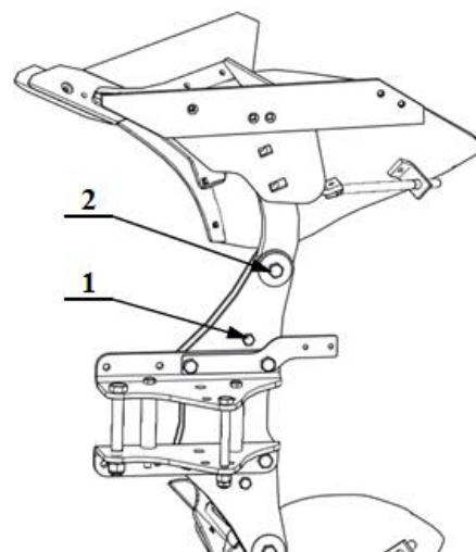
Rysunek:11 Bezpiecznik
