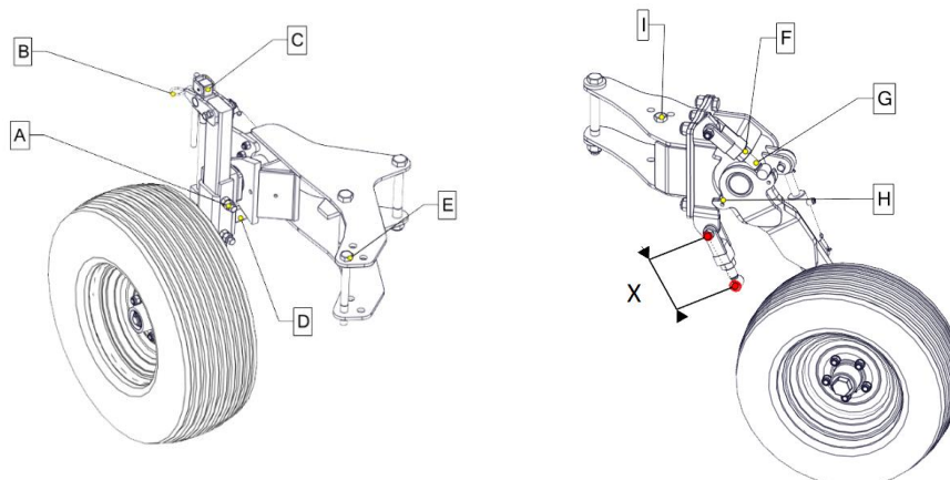
Rysunek:14 Koło podporowe
