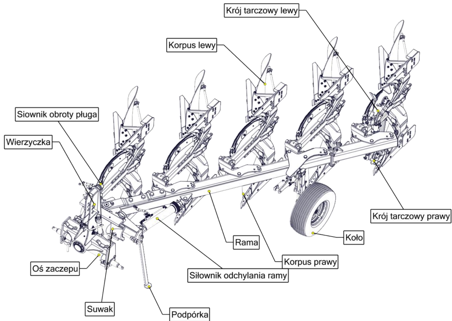
Rysunek:2 Identyfikacja maszyny
