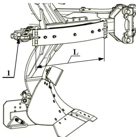
Rysunek:12 Resor
