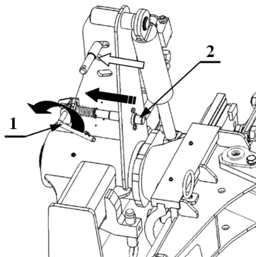
Rysunek:16 Blokada
