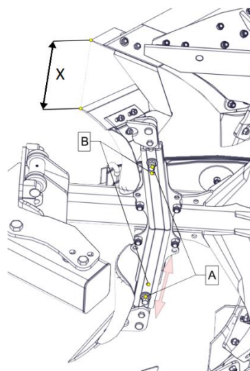
Rysunek:9 Przedpłużek
