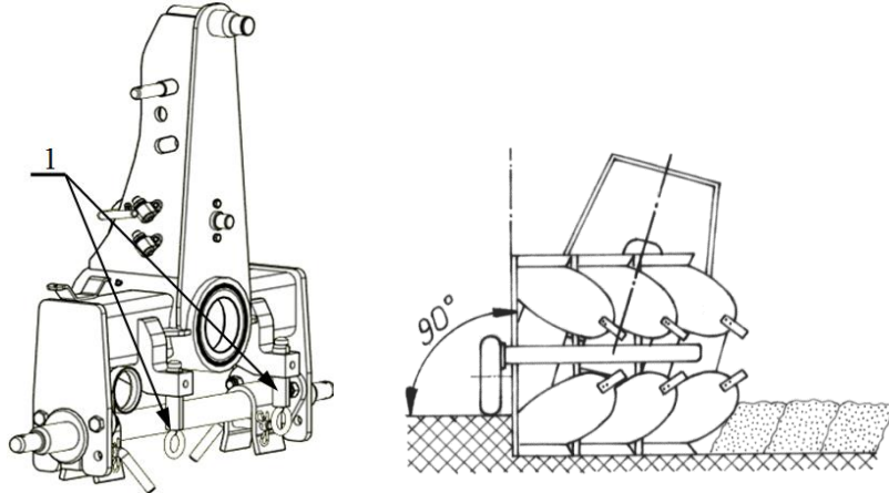
Rysunek:19 Śruby zderzakowe
