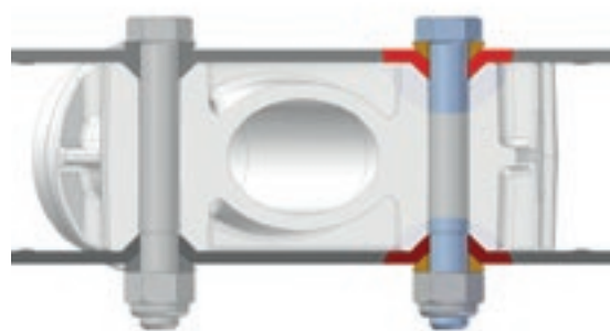
Mocowanie śrubowe z pierścieniami stożkowymi
