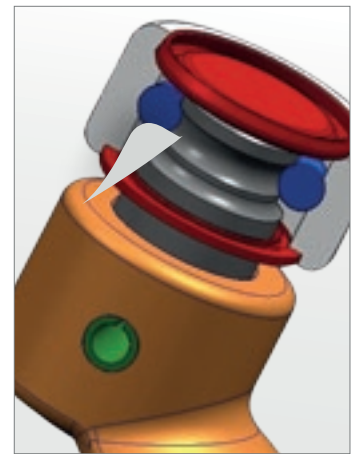
Smarowane dożywotnio, stalowe rolki bieżne na łożyskach kulkowych
