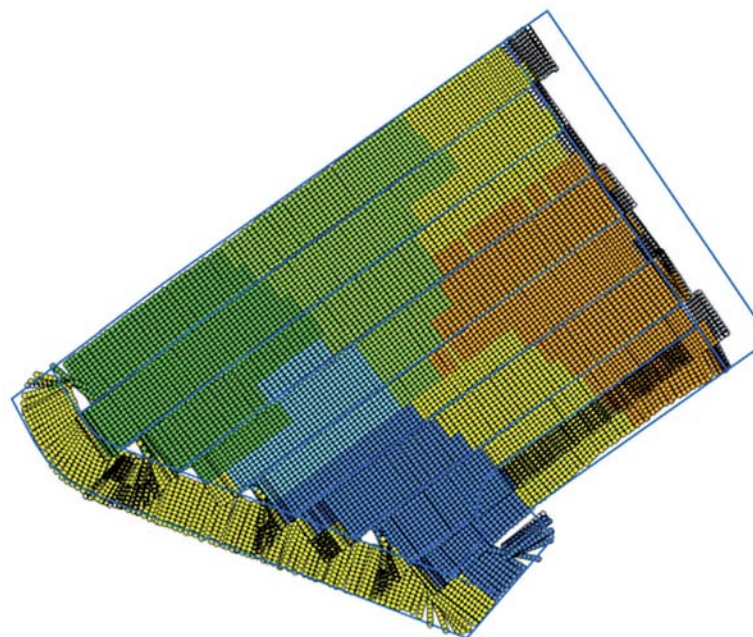
Uzyskana mapa (ekstremalnie bliska rzeczywistości) po rozsiewie nawozu z systemem zmiennego dawkowania niezależnie na prawą/lewą stronę z wykorzystaniem sygnału GPS
